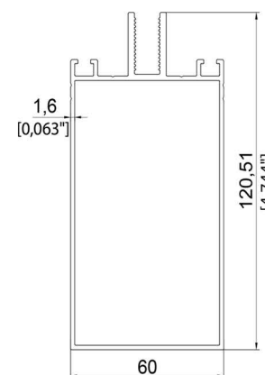
montant
