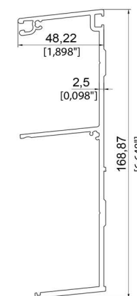
profil perete
