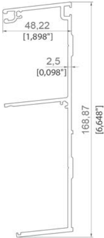
3053 2,250 KG/M
