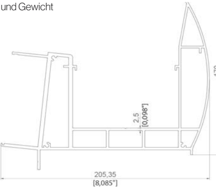
3536 7,095 KG/M
