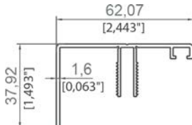
3044 0,640 KG/M
