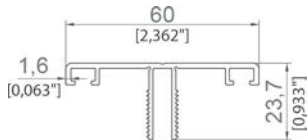
3045 0,520 KG/M
