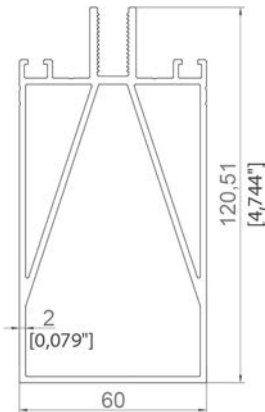
3046 2,920 KG/M
