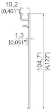
2489 0,458 KG/M
